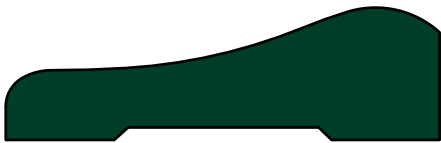
RM 321* 11/16 x 2 1/4
