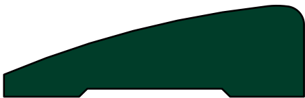
RM 316* 11/16 x 2 1/4
