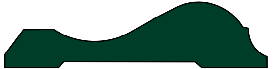
RM 388 11/16 x 2 3/4
